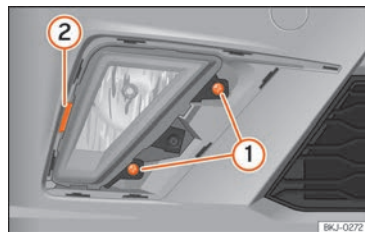
Abb. 165 Nebelscheinwerfer: Lampenträger ausbauen
