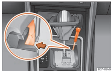
Abb. 92 Wählhebel: Notentriegeln aus der Parkstellung
