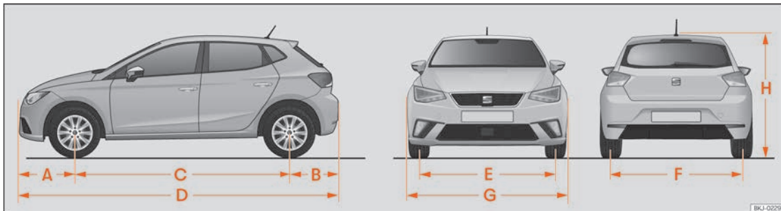
Abb. 194 Abmessungen
