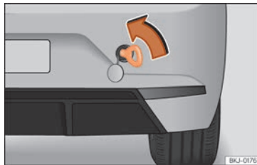
Abb. 158 Auf der rechten Seite des hinteren Stoßfängers: Eingeschraubte Abschleppöse.
