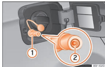
Abb. 147 Geöffnete Tankklappe: Gas-Einfüllstutzen ①, Dichtring des Einfüllstutzens ②.
