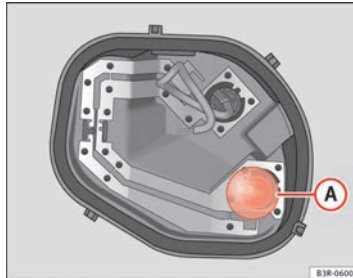
Abb. 227 Position der Glühlampen am Lampenträger: Beispiel: Linke äußere Heckleuchte.
