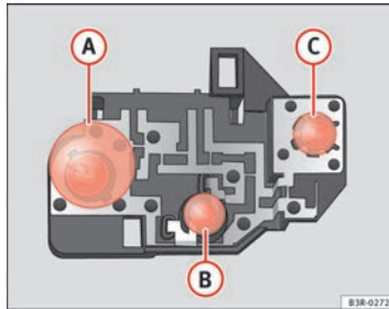
Abb. 235 Position der Glühlampen am Lampenträger. Beispiel: Heckleuchte in der Gepäckraumklappe
