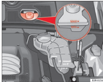
Abb. 188 Motorraum: Markierungen am Bremsflüssigkeitsbehälter
