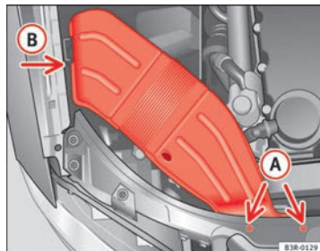
Abb. 217 Luftführungshutze an rechter Fahrzeugseite
