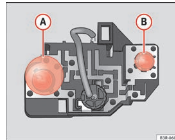
Abb. 236 Position der Glühlampen am Lampenträger. Beispiel: Heckleuchte in der Gepäckraumklappe
