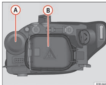
Abb. 218 Glühlampen für Bi-Xenon-Scheinwerfer AFS
