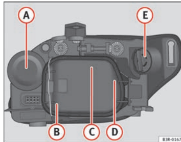
Abb. 206 Glühlampen des Halogenscheinwerfers
