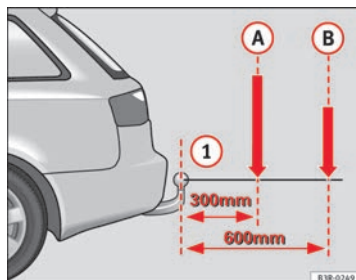
Abb. 164 Prinzipdarstellung der Lastverteilung von Anbauteilen und Zubehör
