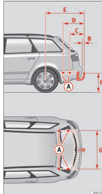
Abb. 175 Befestigungspunkte für die Anhängervorrichtung
