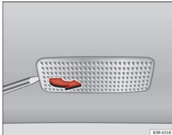
Abb. 242 Ausbau der Leuchte in der Sonnenblende
