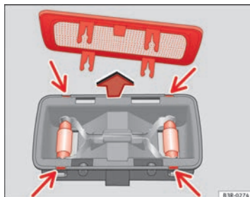
Abb. 239 Gepäckraum- beleuchtung
