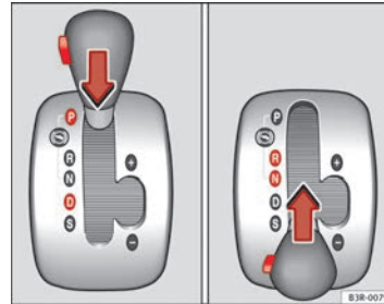
Abb. 159 Wählhebelsperre
