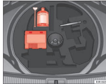
Abb. 194 Reifenreparaturset (Tire-Mobility-System) unter Ladeboden im Gepäckraum
