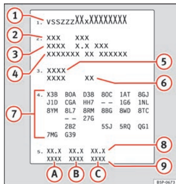
Abb. 247 Fahrzeugdatenträger (Gepäckraum)
