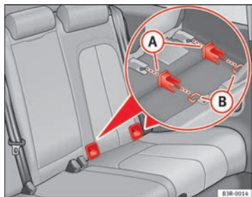
Abb. 32 Lage der ISOFIX-Verankerungen am äußeren Rücksitz
