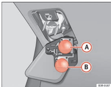
Abb. 217 Position der Glühlampen am Lampenträger. Beispiel: Heckleuchte in der Gepäckraumklappe
