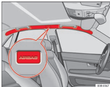
Abb. 25 Einbaulage der Kopfairbags auf der linken Fahrzeugseite
