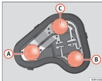
Abb. 209 Position der Glühlampen am Lampenträger. Beispiel: linke Heckleuchte im Kotflügel.
