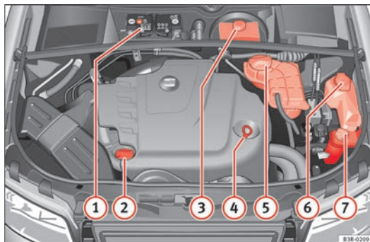
Abb. 229 Abbildung für die Einbaustellen der Elemente
