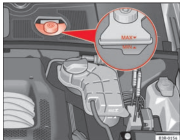
Abb. 172 Motorraum: Markierungen am Bremsflüssigkeitsbehälter
