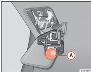
Abb. 218 Position der Glühlampe am Lampenträger. Beispiel: Heckleuchte in der Gepäckraumklappe
