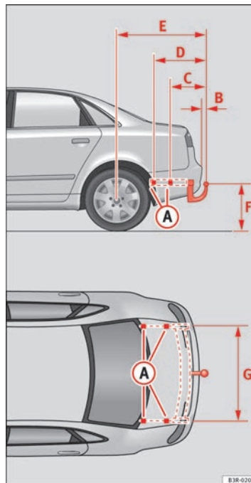
Abb. 161 Befestigungspunkte für die Anhangevorrichtung
