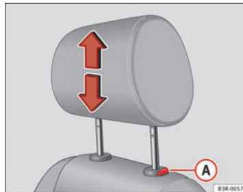
Abb. 111 Vordersitze: Kopfstützen ▶
