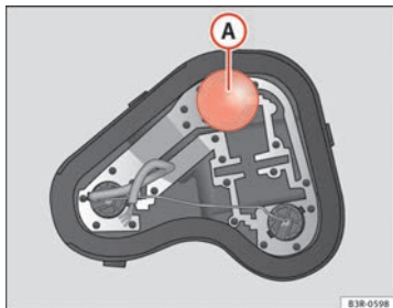
Abb. 210 Position der Glühlampe am Lampenträger. Beispiel: linke Heckleuchte im Kotflügel.
