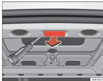
Abb. 224 Gepäckraumbeleuchtung
