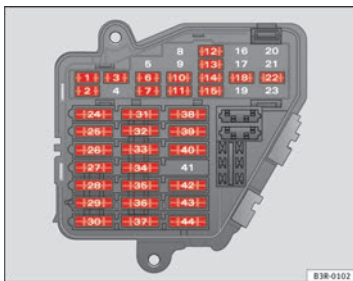
Abb. 191 Prinzipielle Abbildung des Sicherungsträgers an der linken Stirnseite der Schalttafel: Sicherungen (ohne Sicherungsdeckel) ▶
