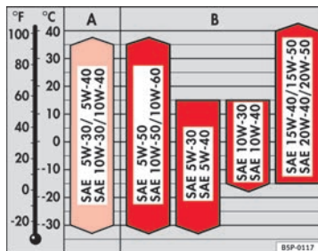
Abb. 169 Öltypen nach Temperaturbereichen
