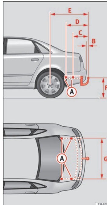
Abb. 163 Befestigungspunkte für die Anhangevorrichtung
