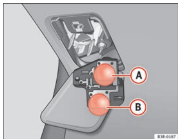
Abb. 222 Position der Glühlampen am Lampenträger. Z.B.: Heckleuchte in der Heckklappe
