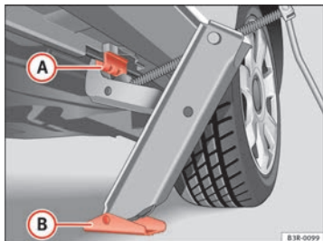
Abb. 185 Radwechsel: Wagenheber
