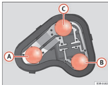
Abb. 216 Position der Glühlampen am Lampenträger: Z.B.: linke Heckleuchte im Kotflügel.
