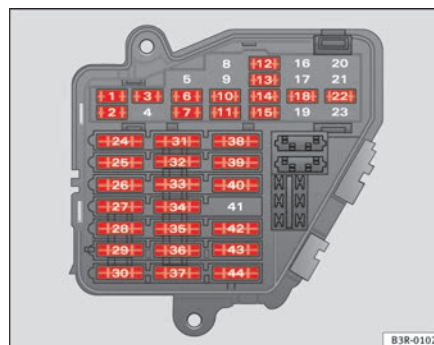
Abb. 186 Prinzipielle Abbildung des Sicherungsträgers an der linken Stirnseite der Schalttafel: Sicherungen (ohne Sicherungsdeckel)
