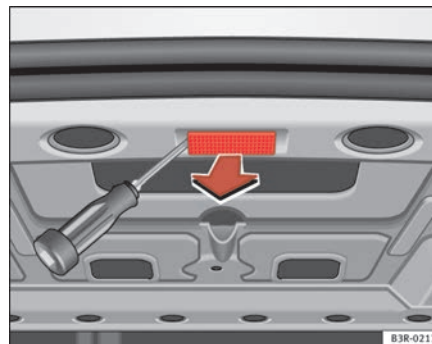
Abb. 219 Gepäckraumbeleuchtung
