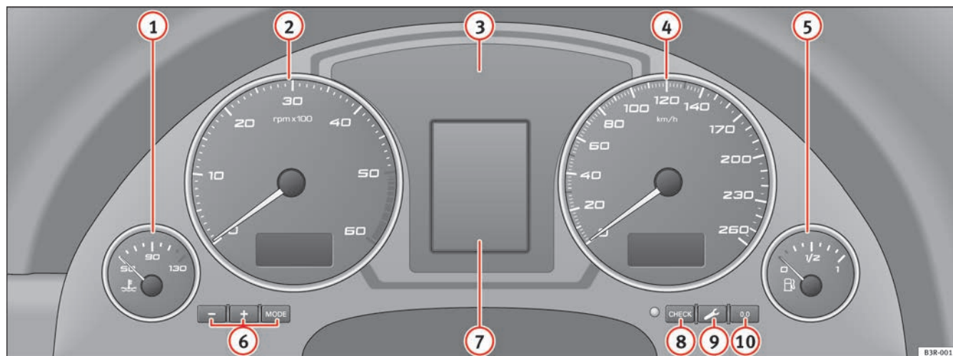
Abb. 37 Übersicht Kombiinstrument
