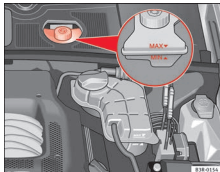
Abb. 171 Motorraum: Markierungen am Bremsflüssigkeitsbehälter
