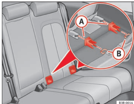
Abb. 32 Lage der ISOFIX-Verankerungen am äußeren Rücksitz
