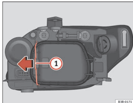
Abb. 195 Standlicht (Fahrzeugaußenseite)
