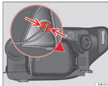
Abb. 196 Standlicht (Fahrzeugaußenseite)
