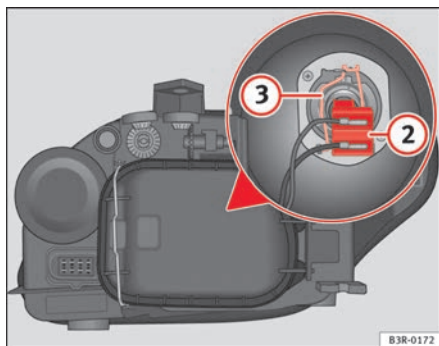
Abb. 194 Abblendlicht
