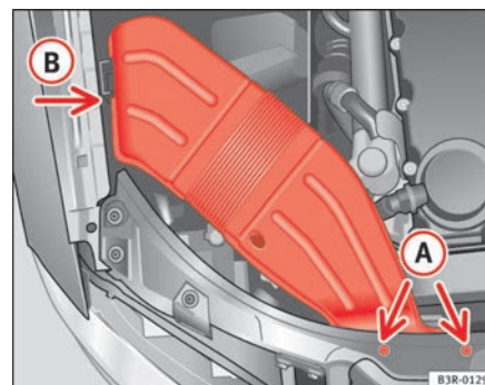
Abb. 200 Luftführungshutze an rechter Fahrzeugseite
