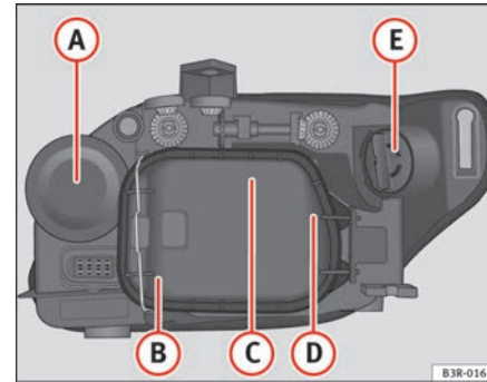
Abb. 189 Glühlampen des Halogenscheinwerfers
