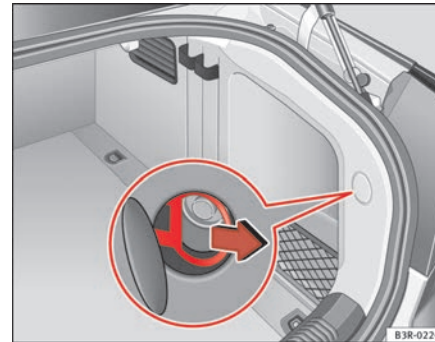
Abb. 161 Gepäckraum: Notentriegeln der Tankklappe
