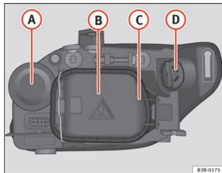
Abb. 201 Glühlampen für Bi-Xenon-Scheinwerfer AFS
