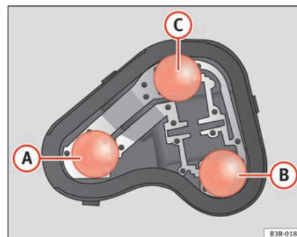
Abb. 211 Position der Glühlampen am Lampenträger: Z.B.: linke Heckleuchte im Seitenteil.
