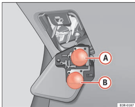
Abb. 217 Position der Glühlampen am Lampenträger. Z.B.: Heckleuchte in der Heckklappe
