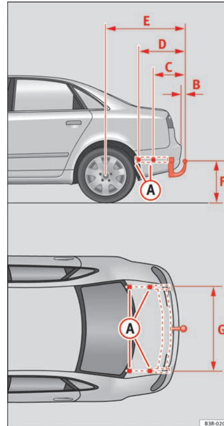
Abb. 158 Befestigungspunkte für die Anhängervorrichtung
