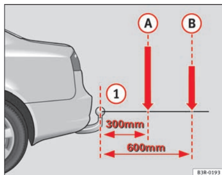
Abb. 147 Prinzipdarstellung der Lastverteilung von Anbauteilen und Zubehör
