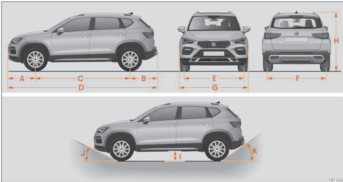
Abb. 225 Abmessungen
