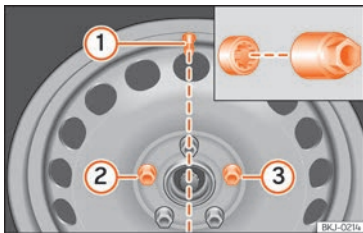
Abb. 220 Radwechsel: Reifenventil ① und Einbauort der Anti-Diebstahl-Radschraube ② oder ③.
