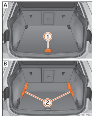
Abb. 168 Variabler Gepäckraumboden: A Hochstellung; B Tiefstellung.
