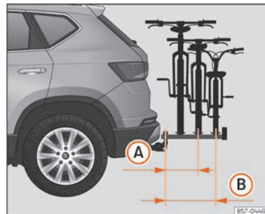
Abb. 181 Schematische Darstellung des maximalen Überstands der Ladung in einem Fahrradträger für zwei oder drei Fahrräder.
