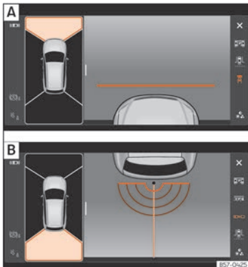
Abb. 146 Bildschirmanzeige der Rundumsicht: A Vordere Kamera: Geländeansicht. B Hintere Kamera: Geländeansicht.
