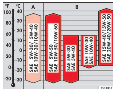
Abb. 159 Öltypen nach Temperaturbereichen
