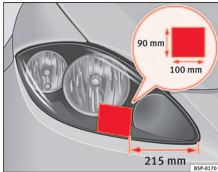
Abb. 150 Rechter Scheinwerfer
