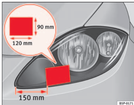
Abb. 151 Linker Scheinwerfer
