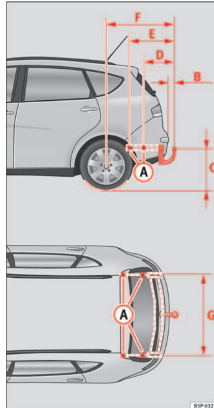
Abb. 155 Befestigungspunkte für die Anhangvorrichtung
