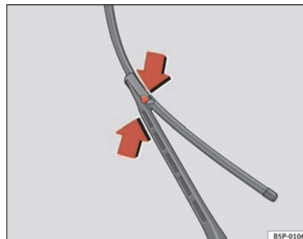
Abb. 165 Scheibenwischerblätter vorne austauschen
