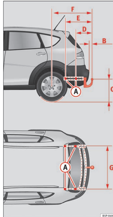
Abb. 153 Befestigungspunkte für die Anhangervorrichtung
