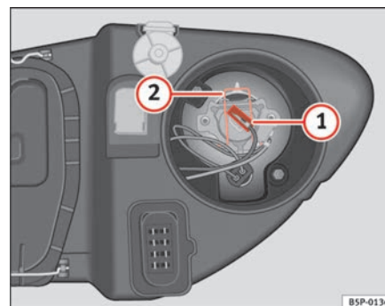
Abb. 184 Fernlicht
