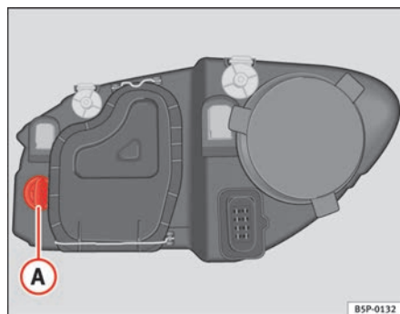
Abb. 180 Glühlampe für Blinker
