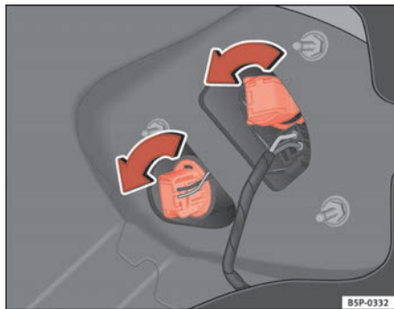
Abb. 188 Rücklichter an der Karosserie
