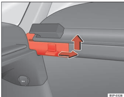
Abb. 124 Die Ablage ausbauen
