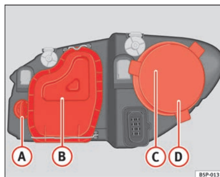
Abb. 179 Glühlampen des Hauptscheinwerfers ►
