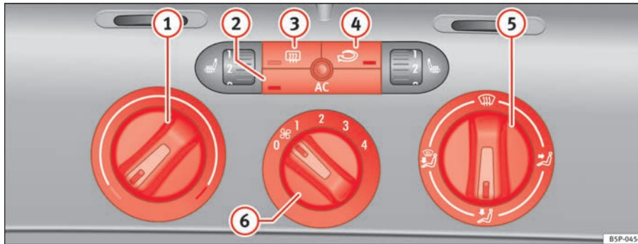
Abb. 130 In der Instrumententafel: Bedienelemente der Climatic
