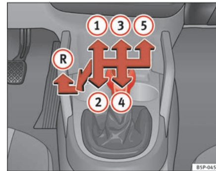
Abb. 139 In der Mittelkonsole: Schaltschema eines 5-Gang-Schaltgetriebes
