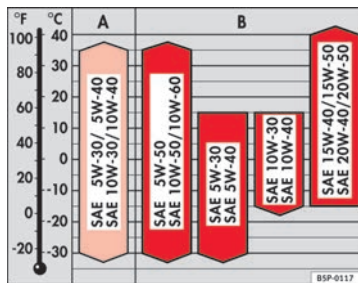
Abb. 157 Öltypen nach Temperaturbereichen
