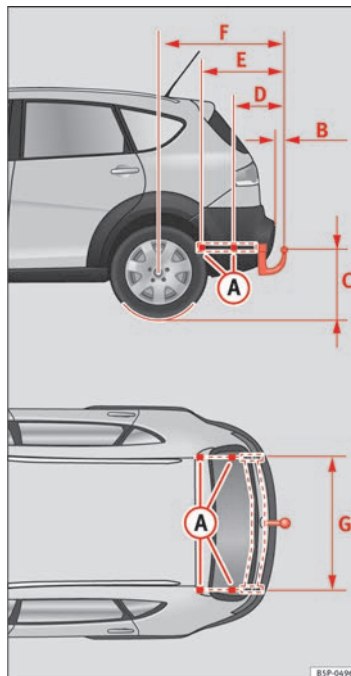
Abb. 153 Befestigungspunkte für die Anhangervorrichtung
