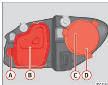
Abb. 182 Glühlampen des Hauptscheinwerfers
