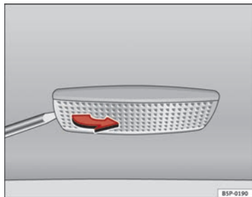
Abb. 200 Ausbau der Leuchte in der Sonnenblende
