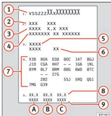
Abb. 206 Fahrzeugdatenträger (Gepäckraum)
