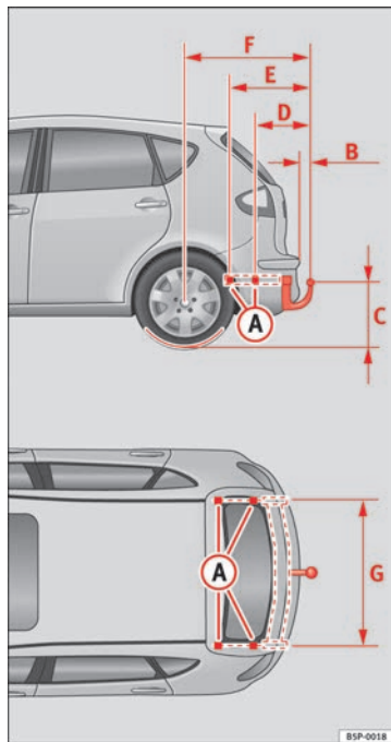
Abb. 156 Befestigungspunkte für die Anhängervorrichtung
