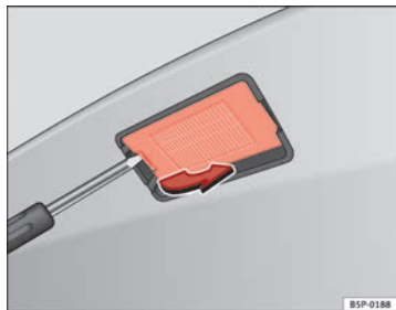
Abb. 198 Kennzeichenbeleuchtung
