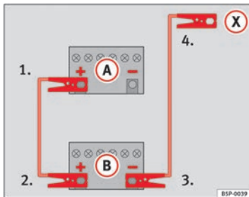
Abb. 202 Schaltschema zum Anschluss der Starthilfekabel, falls das stromgebende Fahrzeug über kein Start-Stopp-System verfügt: entladene Batterie (A) und stromgebende Batterie (B).
