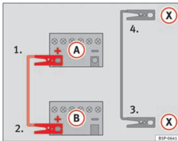
Abb. 203 Schaltschema zum Anschluss der Starthilfekabel, falls das stromgebende Fahrzeug mit einem Start-Stopp-System ausgestattet ist: entladene Batterie (A) und stromgebende Batterie (B).
