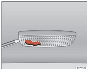
Abb. 201 Ausbau der Leuchte in der Sonnenblende
