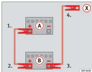
Abb. 203 Anschlussschema der Starthilfekabel, wenn das stromgebende Fahrzeug nicht über das Start-Stopp-System verfügt: entladene Batterie (A) und stromliefernde Batterie (B).
