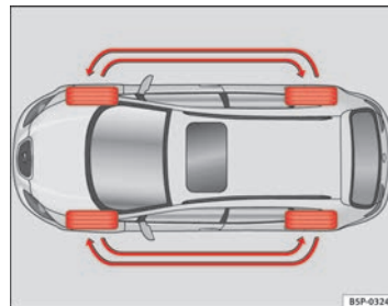
Abb. 173 Schema für das Tauschen der Räder
