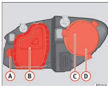
Abb. 183 Glühlampen des Hauptscheinwerfers ▶
