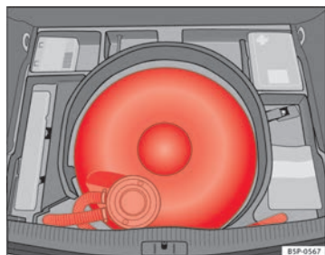
Abb. 159 Autogas-Vorratsbehälter in der Reserveradmulde.
