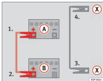
Abb. 204 Anschlussschema der Starthilfekabel, wenn das stromgebende Fahrzeug über das Start-Stopp-System verfügt: entladene Batterie (A) und stromliefernde Batterie (B).
