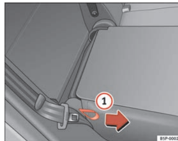
Abb. 99 Umklappen bzw. Aufrechtstellen der Rückenlehne
