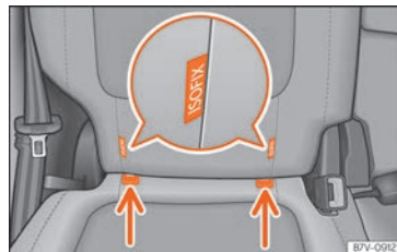
Abb. 29 Rückseite: ISOFIX-Halteösen.
