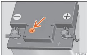
Abb. 293 Sichtfenster an der Oberseite der 12-Volt-Fahrzeuga-batterie (Prinzipdarstellung).
