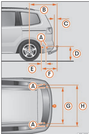
Abb. 279 Maße und Befestigungspunkte für den nachträglichen Einbau einer Anhängervorrichtung
