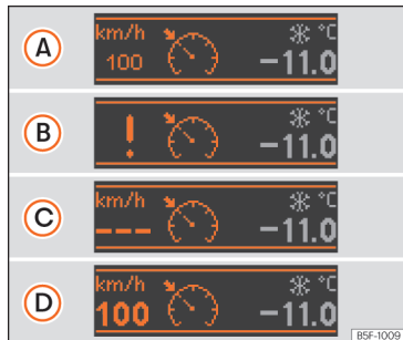
Abb. 247 Bildschirm des Kombi-Instruments: Zustandsanzeigen der GRA.
