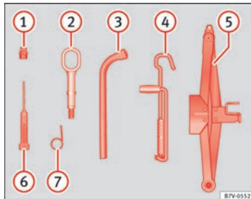
Abb. 200 Bestandteile des Bordwerkzeugs.
