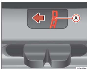
Abb. 194 Vom Gepäckraum aus: Heckklappe notentriegeln.
