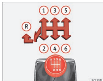
Abb. 131 Schaltschema des 6-Gang-Schaltgetriebes.
