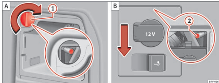
Abb. 213 Seitlich im Gepäckraum: Rückleuchte links und rechts ausbauen. ① Abdeckkappe abziehen, ② Befestigungsschraube.
