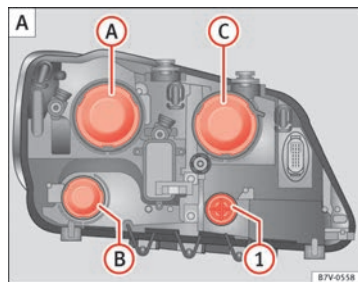
Abb. 205 Im Motorraum: Abdeckungen im linken Frontscheinwerfer. A Abblendlicht, B Tagfahrlicht und C Fernlicht und Standlicht.
