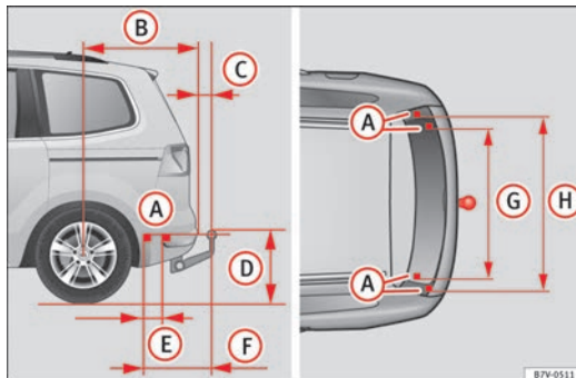
Abb. 159 Maße und Befestigungspunkte zum Nachrüsten einer Anhängervorrichtung.
