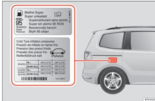
Abb. 178 Einbauort des Reifenfülldruckschildes.
