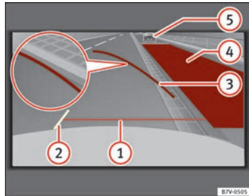
Abb. 150 Im Bildschirm: Orientierungslinien und -flächen des Parkraums hinter dem Fahrzeug.
