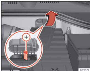
Abb. 217 Im Motorraum: Starthilfepunkt Pluspol (+).
