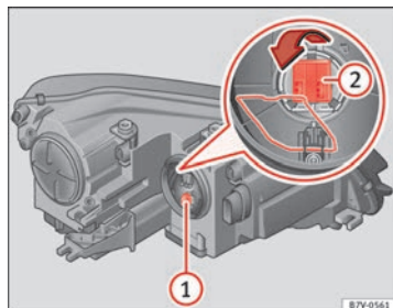
Abb. 208 Blinklichtlam- penhalter ① und Abbie- gelicht ②.
