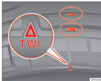
Abb. 179 Reifenprofil: Verschleißanzeiger.
