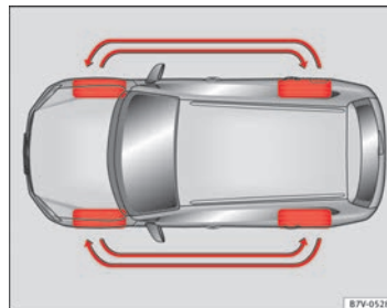
Abb. 177 Schema für das Tauschen der Räder.
