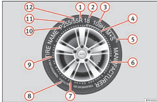
Abb. 180 Internationale Reifenbeschriftung.
