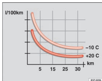
Abb. 157 Kraftstoffverbrauch in l/100 km bei zwei verschiedenen Umgebungstemperaturen.
