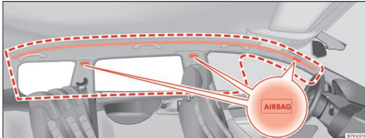
Abb. 22 Auf der linken Fahrzeugseite: Einbauort und Wirkungsbereich des Kopfairbags. ►
