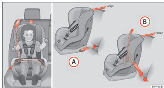
Abb. 26 Auf den Rücksitzen: Abbildung (A) zeigt die prinzipielle Befestigung des Kinderrückhaltesystems an den unteren Halteösen und mit oberem Befestigungsgurt. Abbildung (B) zeigt die Befestigung des Kinderrückhaltesystems mit dem Sicherheitsgurt des Fahrzeugs.
