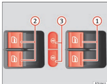
Abb. 56 In der Fahrertür: Tasten für die vorderen und hinteren Fensterheber sowie Tasten für die elektrische Kindersicherung.
