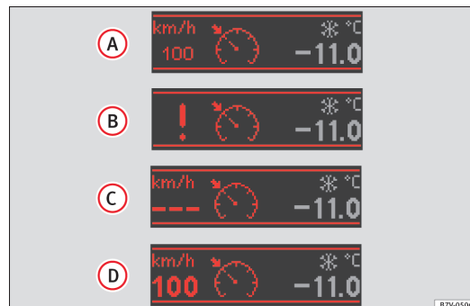
Abb. 151 Im Display des Kombiinstrument: Zustandsanzeigen der GRA.
