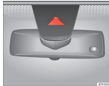
Abb. 153 An der Frontscheibe: Kamerasichtfenster des Spurhalteassistenten.
