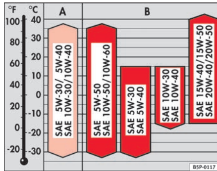
Abb. 140 Öltypen nach Temperaturbereichen
