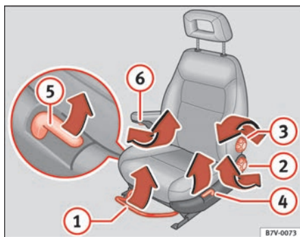
Abb. 86 Bedienelemente am linken Vordersitz
