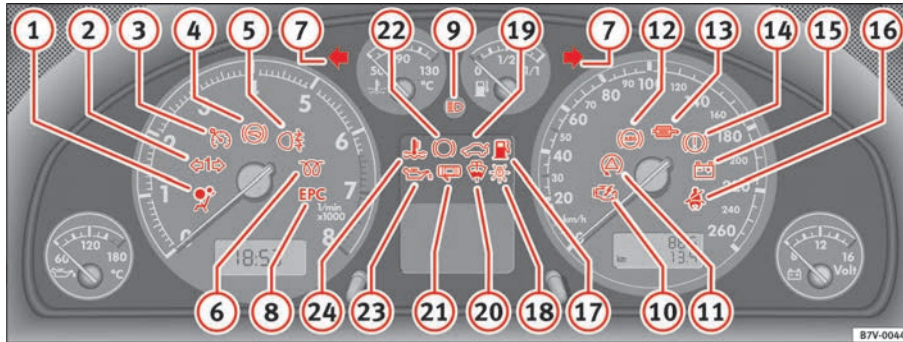
Abb. 48 Kombiinstrument mit Warn- und Kontrollleuchten. Einige der hier aufgeführten Warn- und Kontrollleuchten gehören zu bestimmten Modellausführungen oder sind Bestandteil von Mehrausstattungen.
