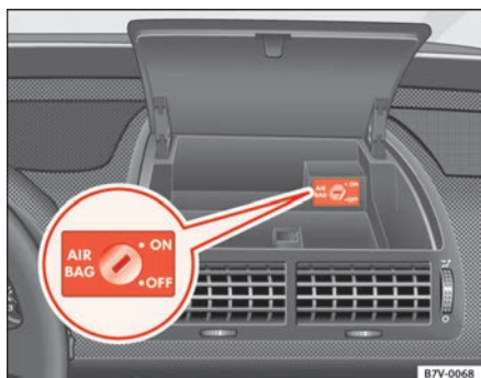
Abb. 28 Innenraum des Ablagefachs in der Mitte der Instrumententafel: Schlüsselschalter zum Abschalten der Beifahrer-Airbags
