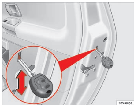
Abb. 59 Hebel für die Kindersicherung in der linken hinteren Tür
