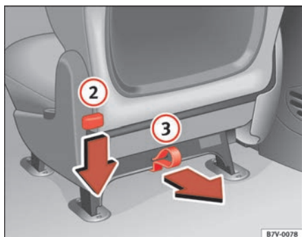
Abb. 91 Rückbereich des Sitzes: Rückenlehne und Sitz vorklappen
