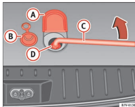
Abb. 152 Reserverad herausnehmen
