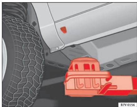
Abb. 174 Anheben mit der Hebebühne: Aufnahmepunkt vorne links
