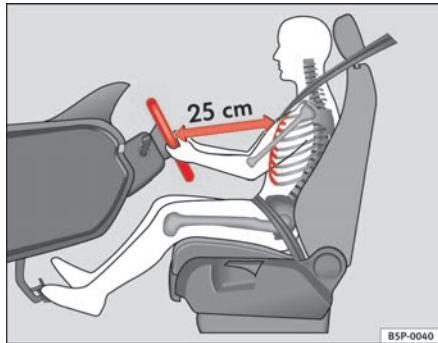
Abb. 122 Lenkradposition einstellen
