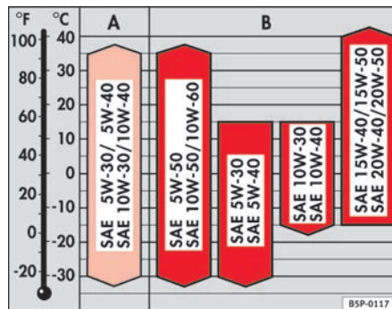
Abb. 139 Öltypen nach Temperaturbereichen
